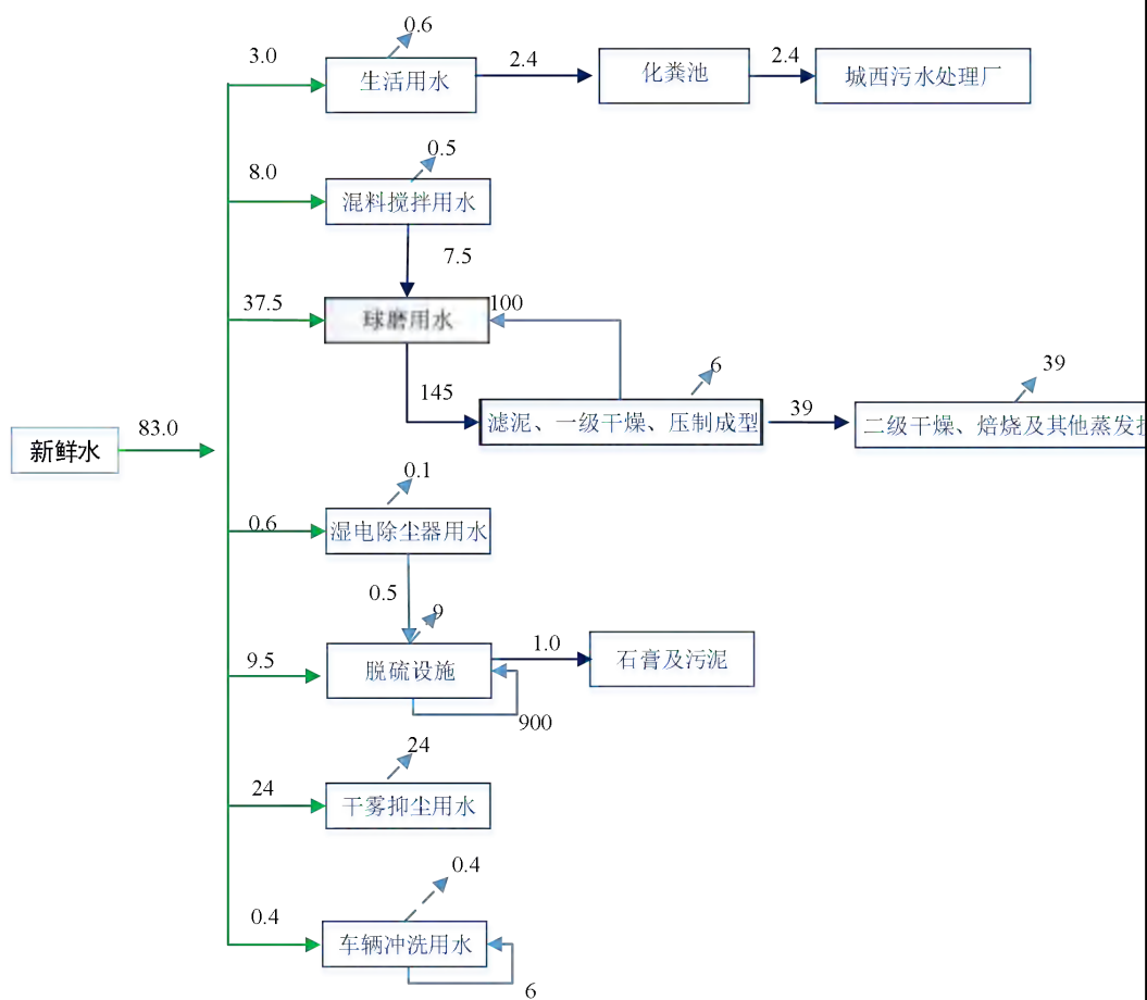
图 2 项目用排水平衡图 m³/d
